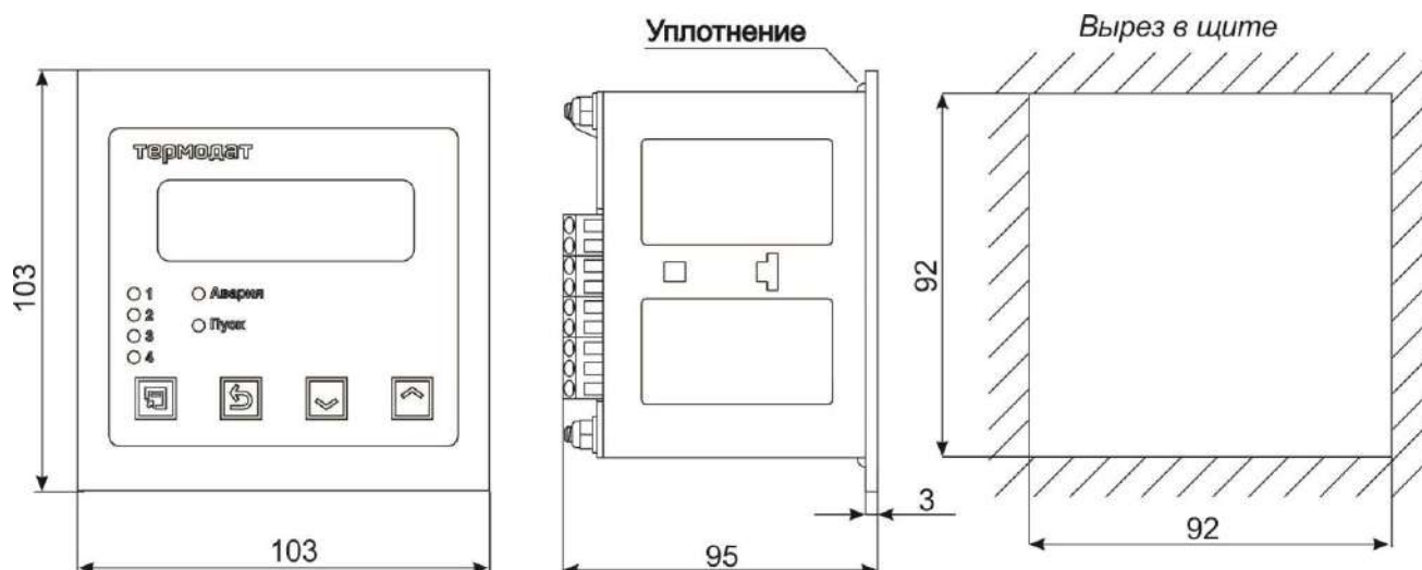
Рисунок 12 – Габаритные размеры прибора Термодат-14Е5/..../IP67пп или Термодат-14Е5-А7
