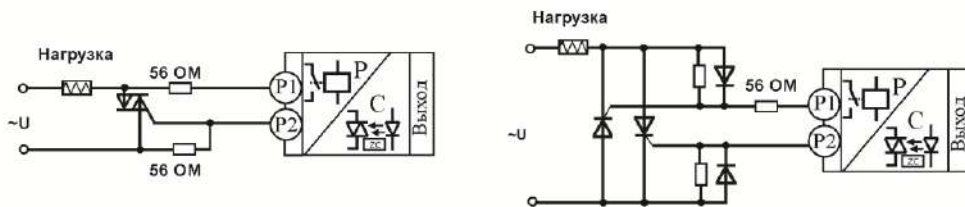
Подключение внешнего симистора
