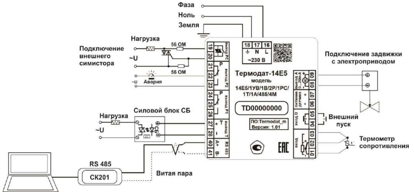
Рисунок 10 – Схема подключения прибора
