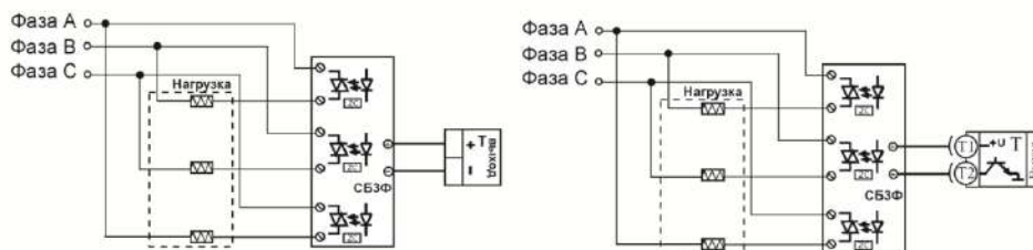
Подключение трехфазной нагрузки в шестипроводной схеме
