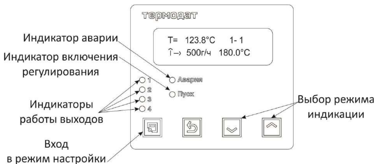
Рисунок 2 – Описание индикаторов и кнопок управления прибора
