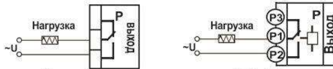
Подключение нагрузки менее 2,3 кВт
