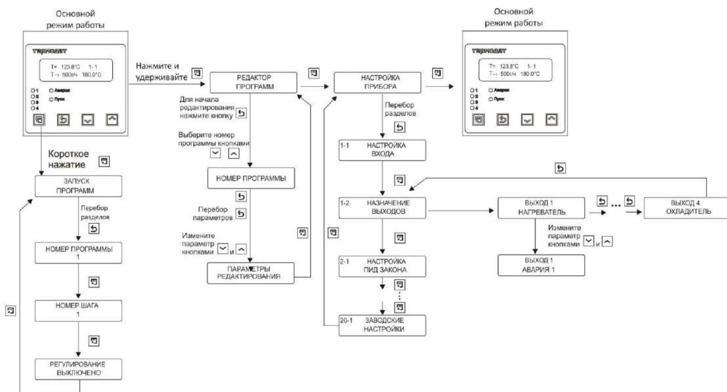
Рисунок 3 – Схема меню
