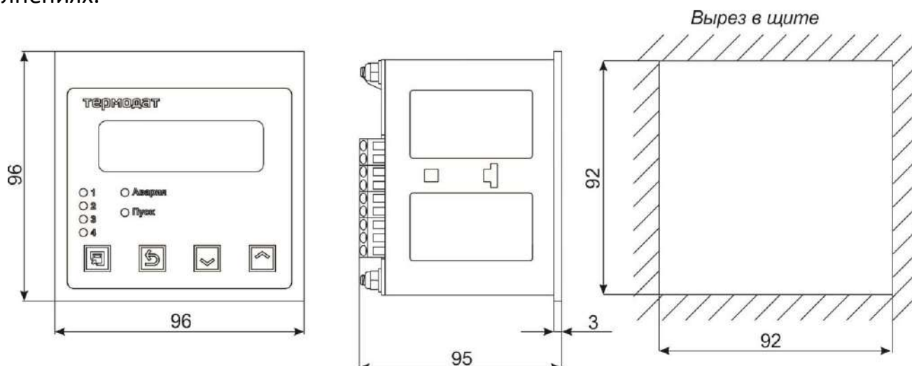
Рисунок 11 – Габаритные размеры прибора 14Е5/..../ или Термодат-14Е5-А
