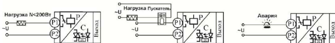
Подключение нагрузки менее 200 Вт
